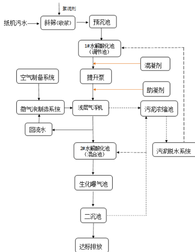
图 2.2-1 厂内污水处理系统工艺流程图
