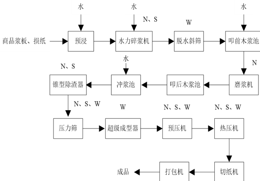
图 2.1-1 厚型绝缘纸板生产线工艺流程及产污环节图
