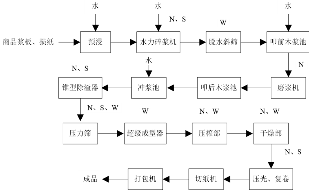
图 2.1-2 薄型绝缘纸板生产线工艺流程及产污环节图
